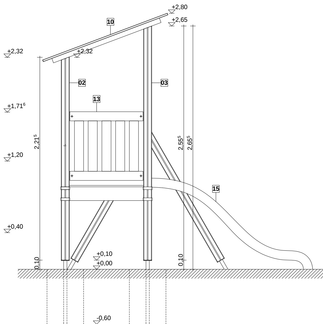
oldalnézet m1:25
