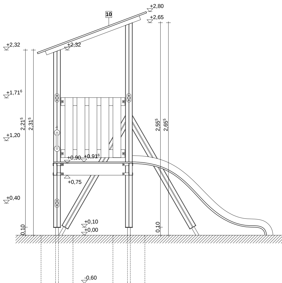
metszet m1:25
