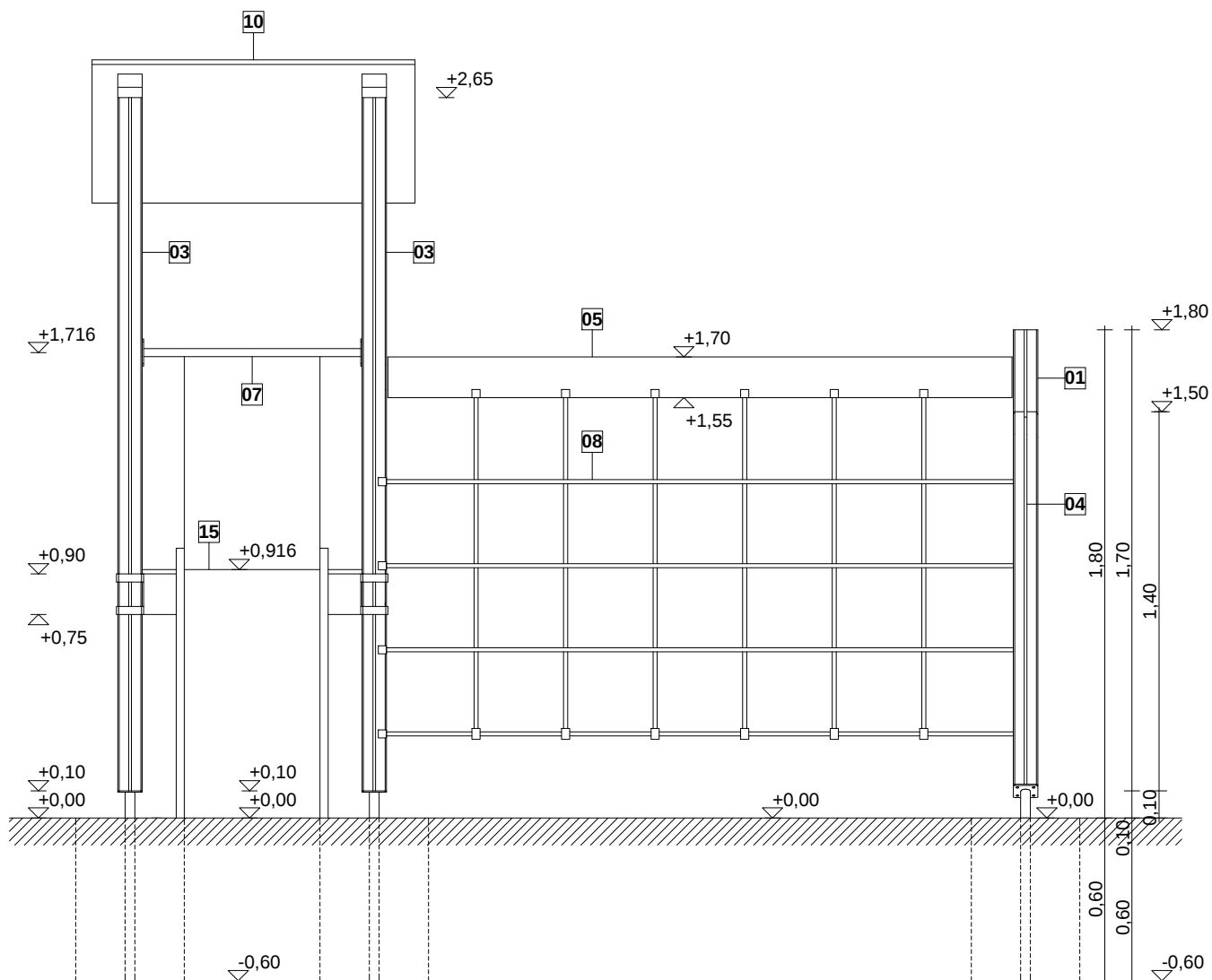
előlnézet m1:25
