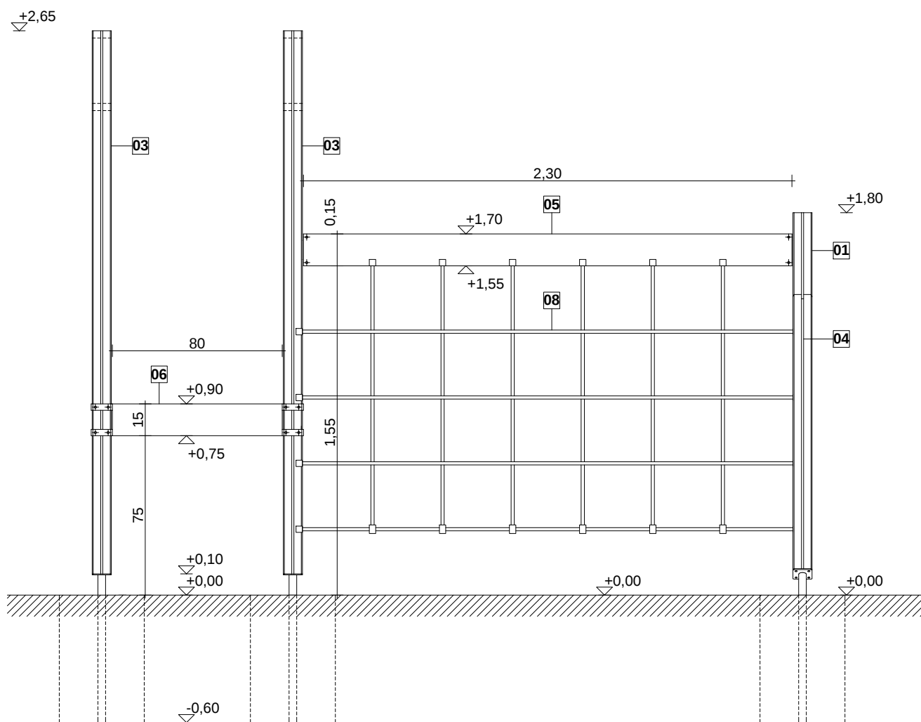
palló szerelési rajz - előlnézet m1:25
