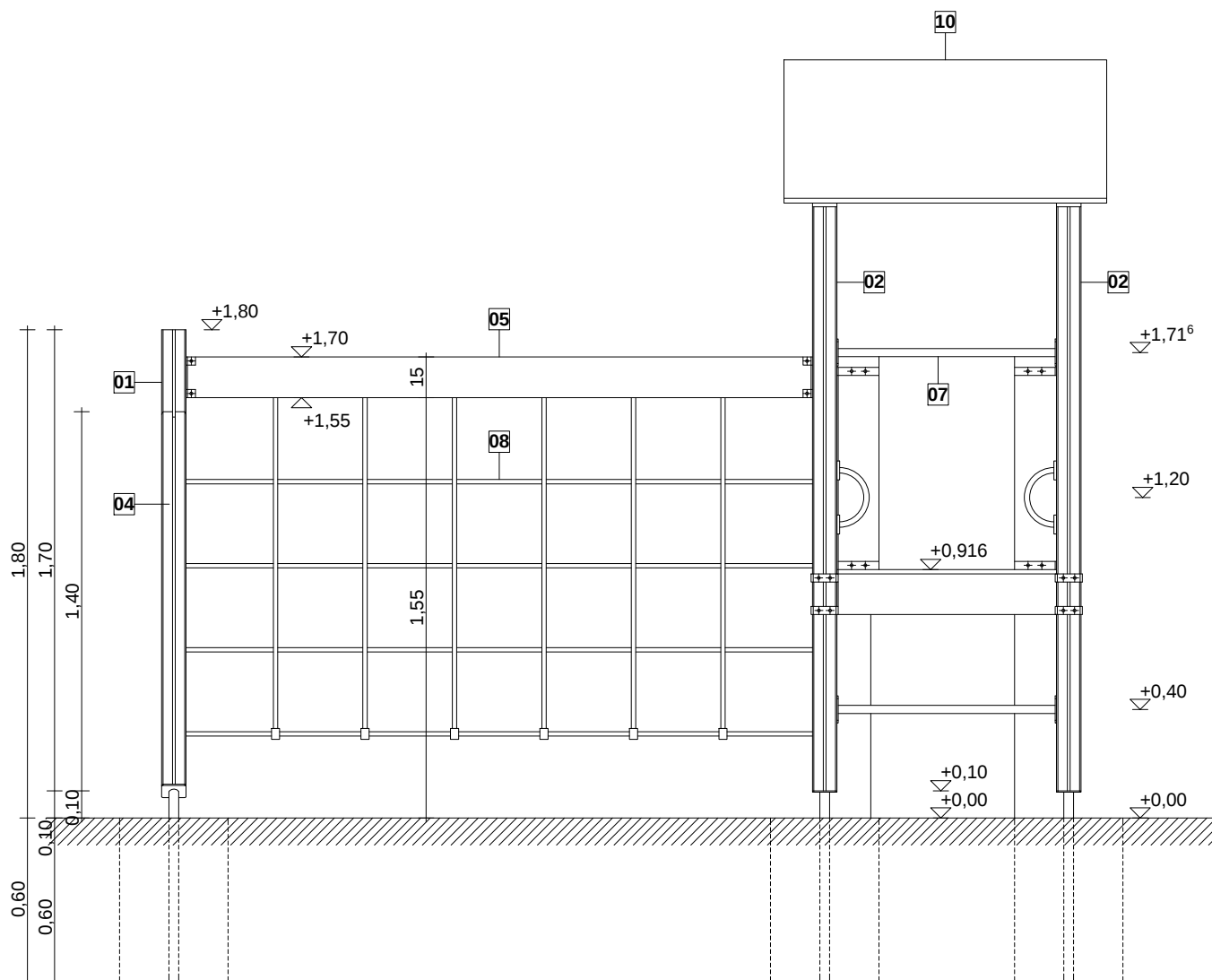
hátnézet m1:25
