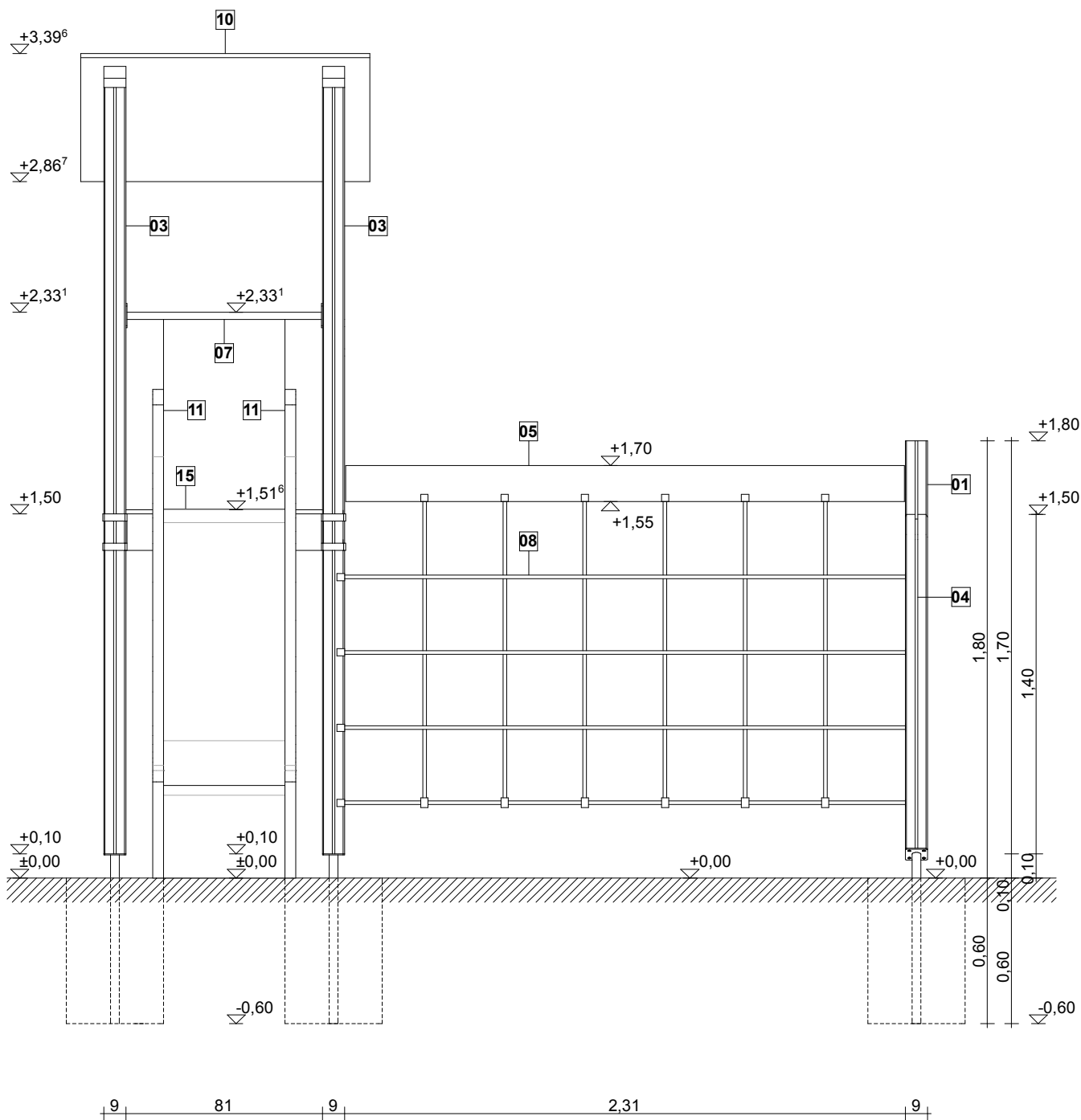
előlnézet m1:25
