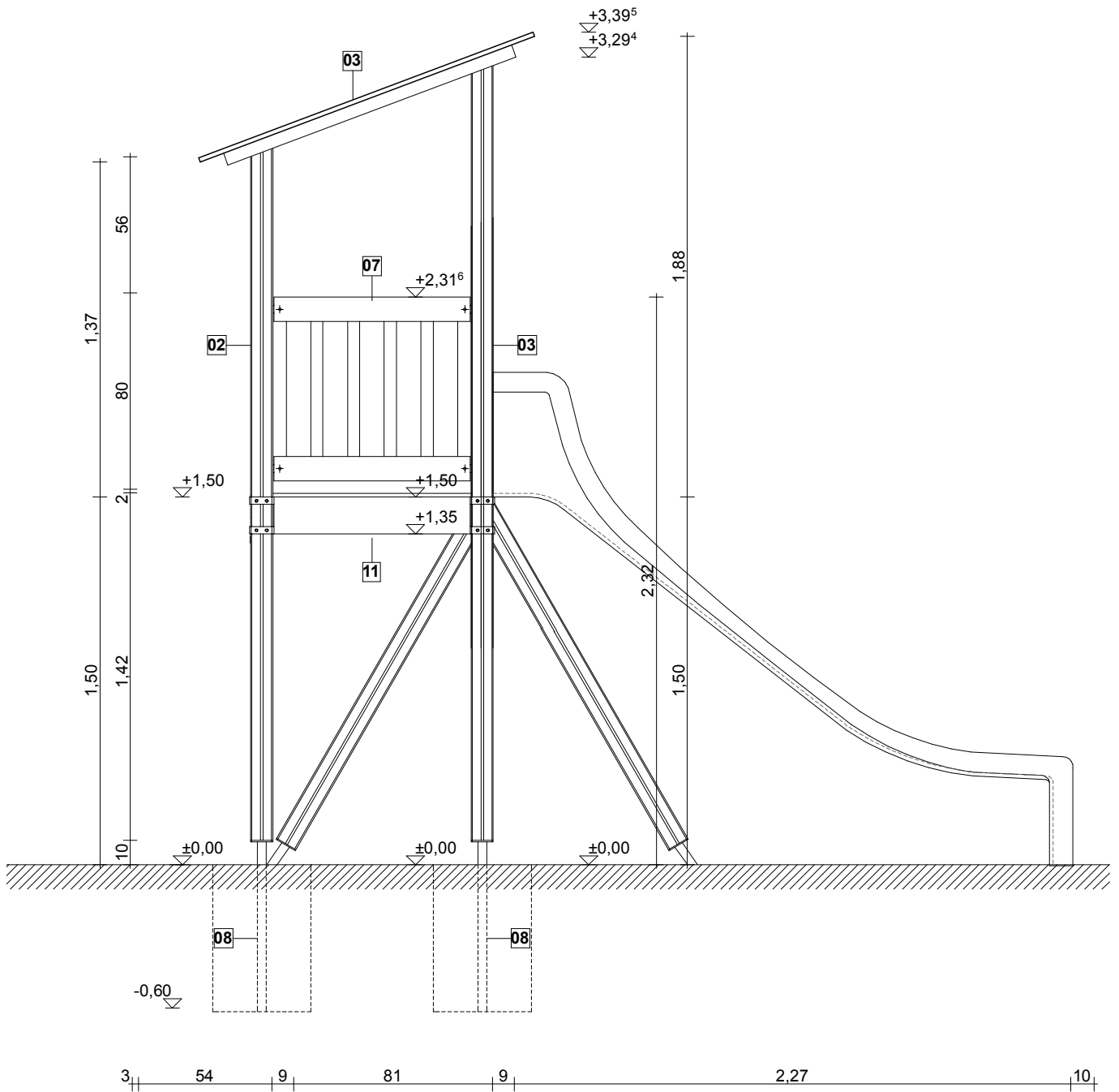
oldalnézet m1:25
