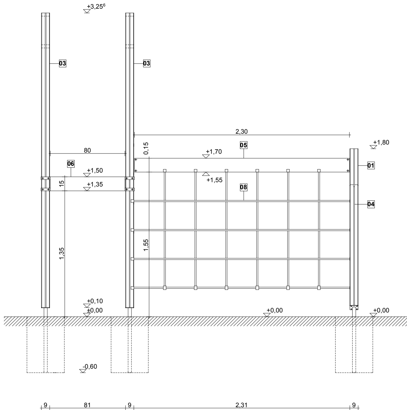
palló szerelési rajz - előlnézet m1:25
