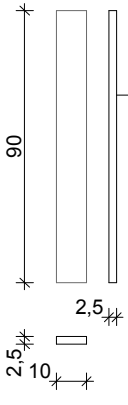
12 jelű 2 5 /10 deszka hossz: 900 mm - 10db
