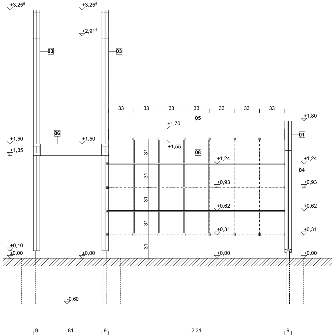
háló szerelési rajz - előlnézet m1:25
