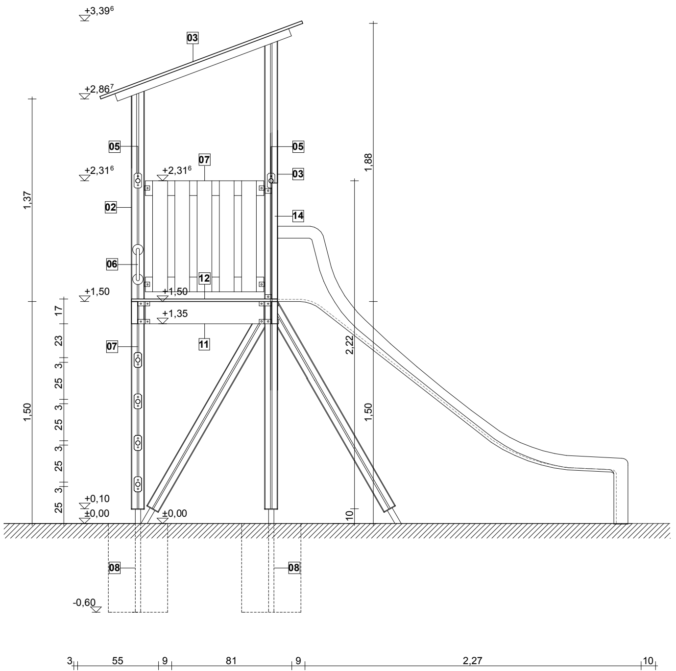
metszet m1:25
