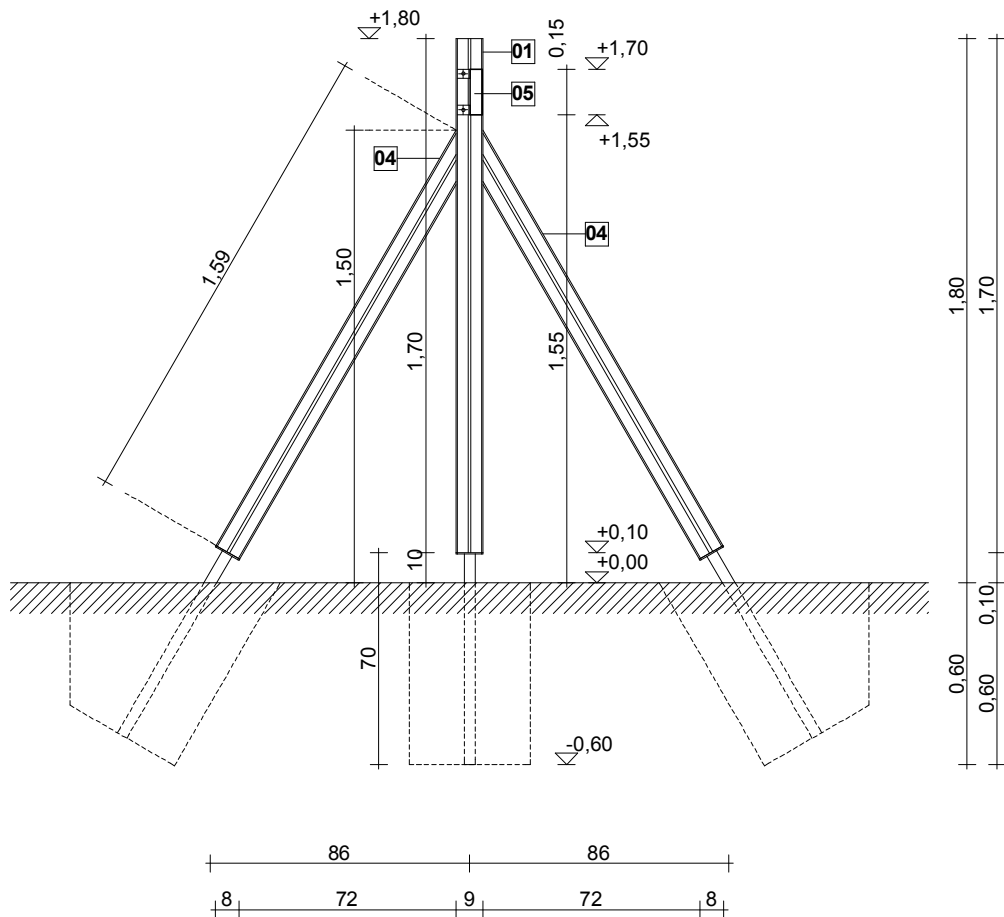
oszlop szerelési rajz - 02_02 jelű metszet m1:25
