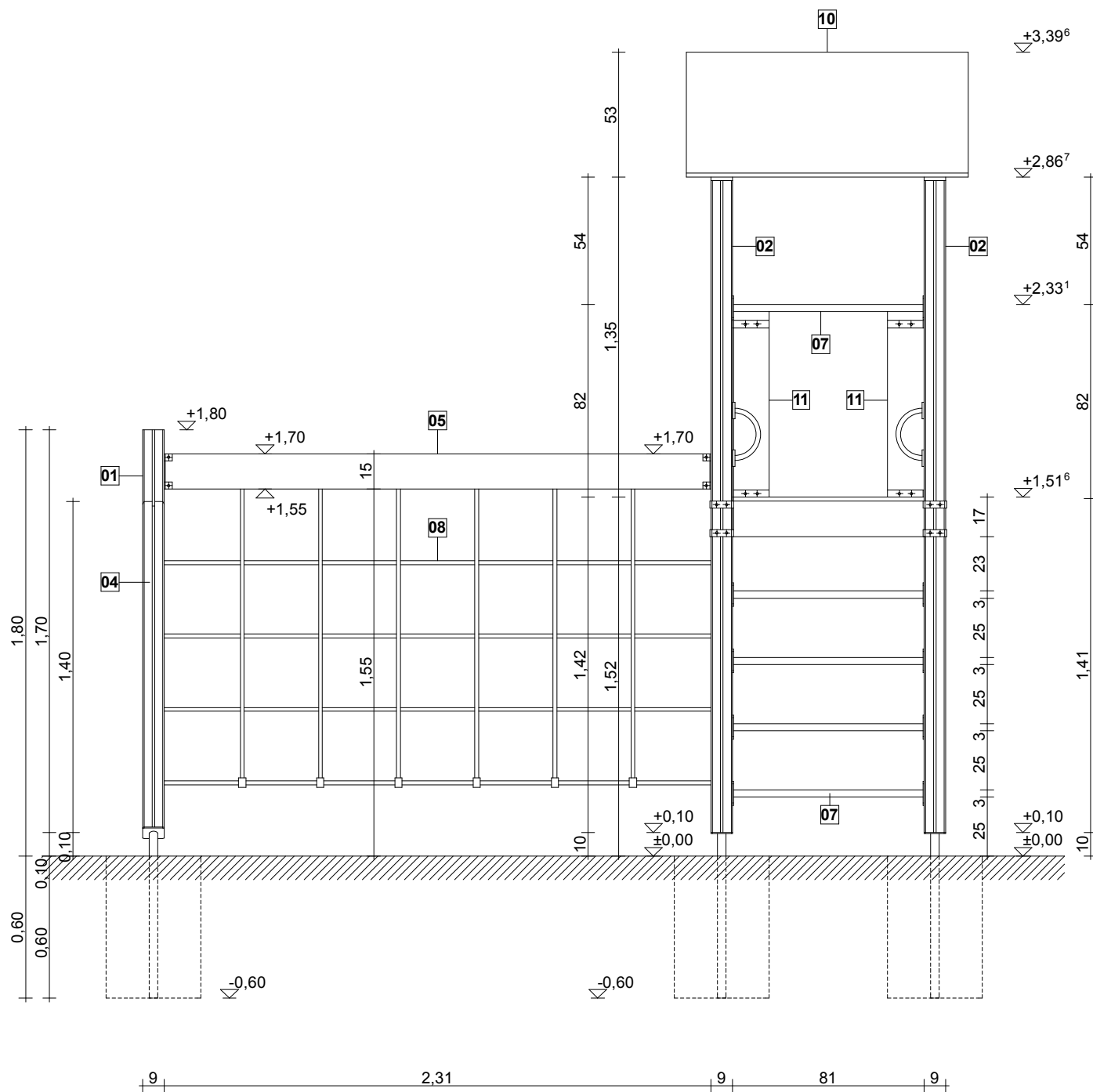
hátulnézet m1:25
