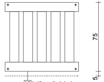
13 jelű mellvéd elem 80 x 75 cm 2 db
