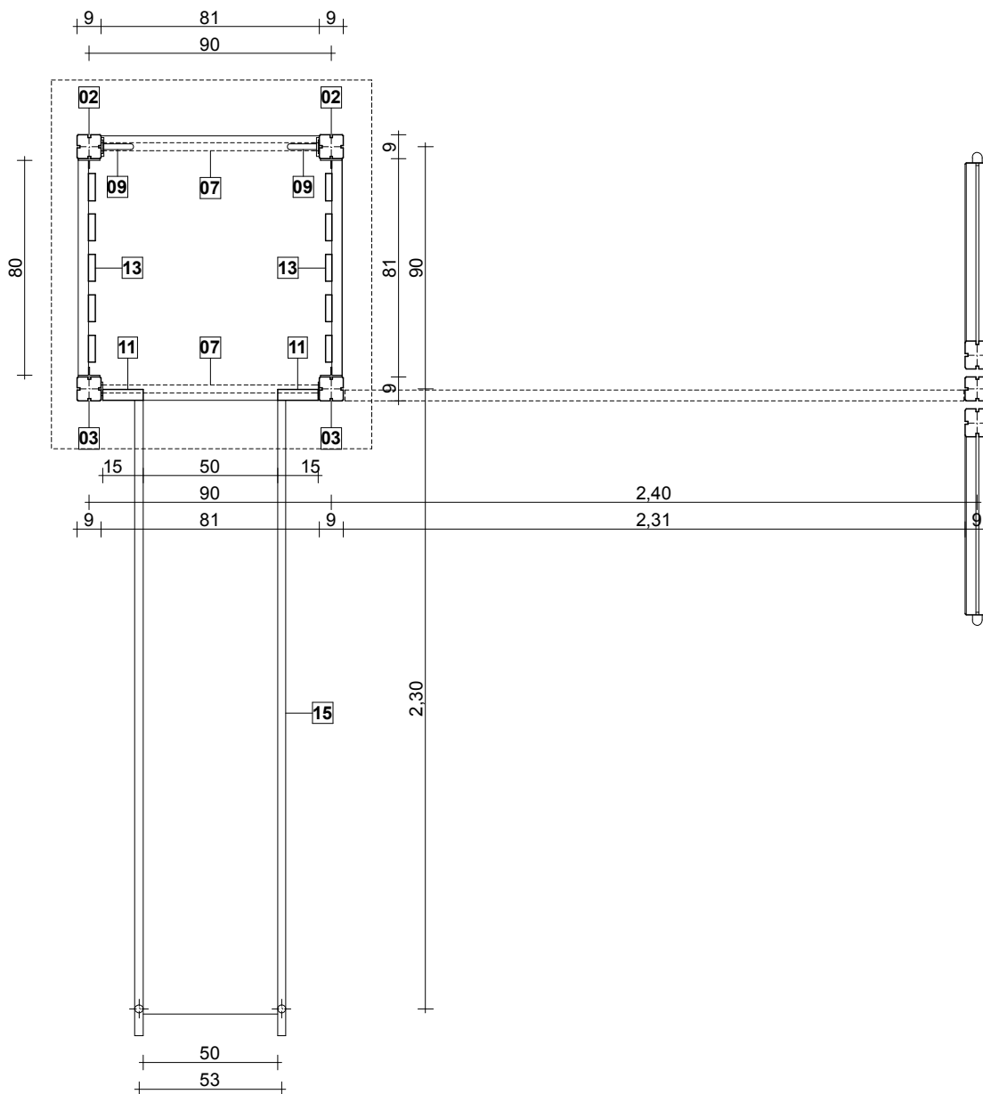
alaprjz / vízszintes metszet +1,25 m / m1:25
