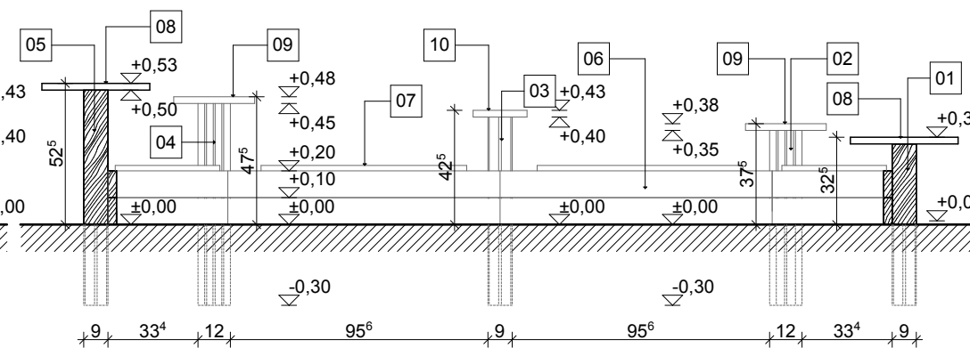
hosszmetszet m1:25
