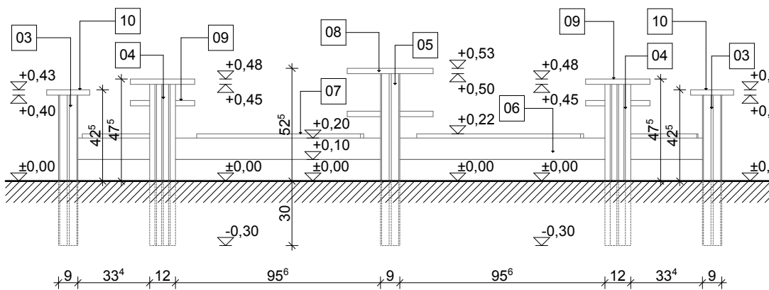
előlnézet m1:25
