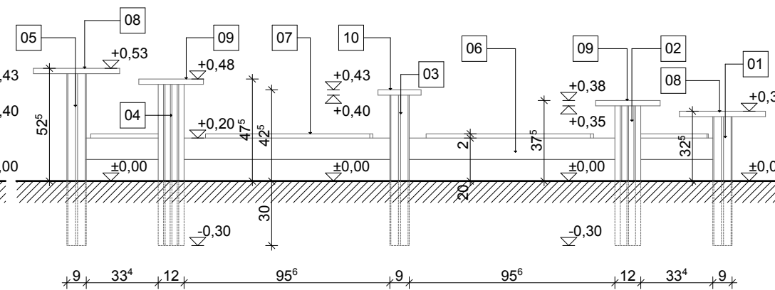
oldalnézet m1:25
