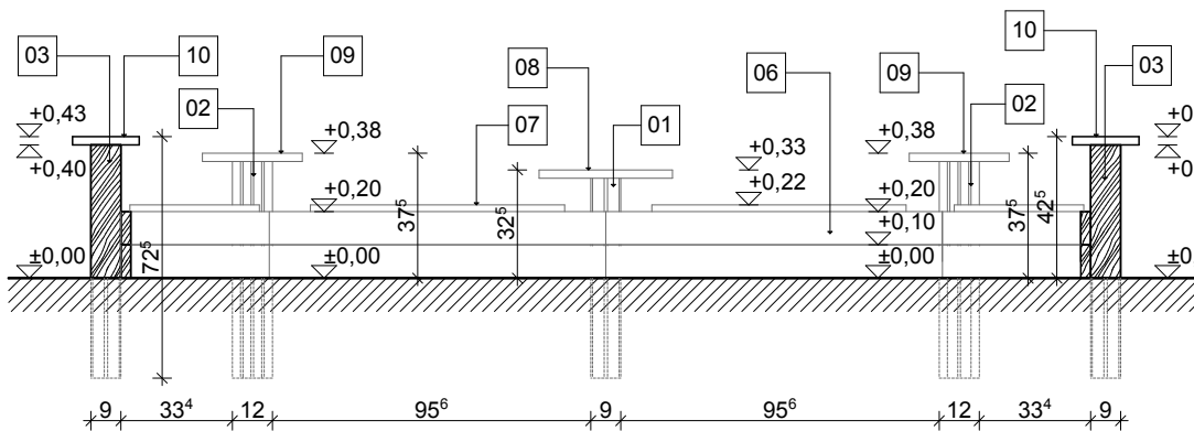
keresztmetszet m1:25
