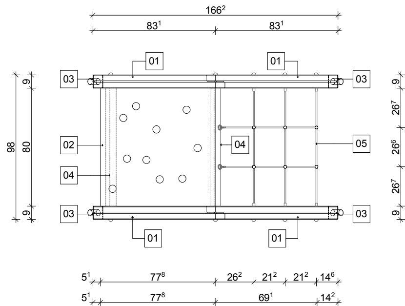
alapozási alaprajz m1:25
