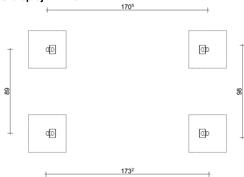
alapozási alaprajz m1:25
