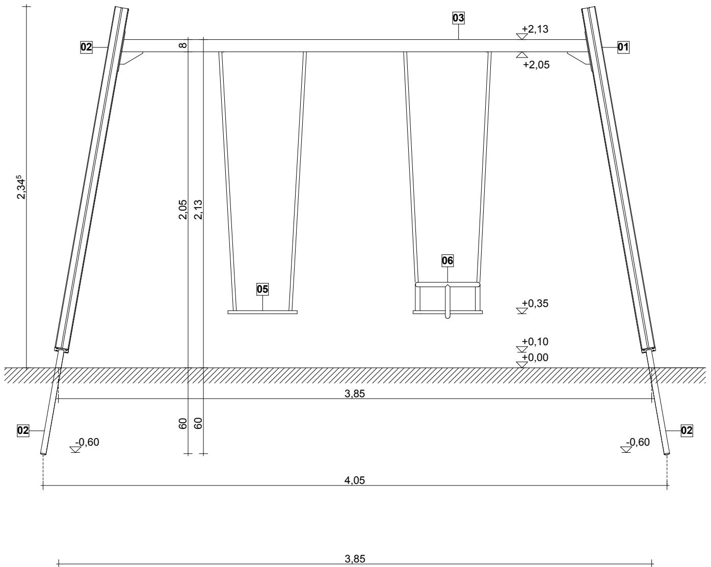
előlnézet m1:25
