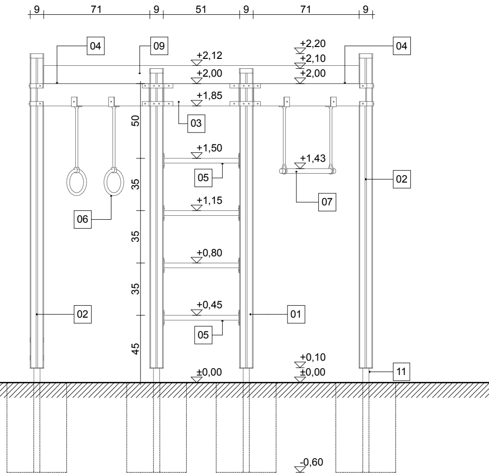
oldalnézet m1:25
