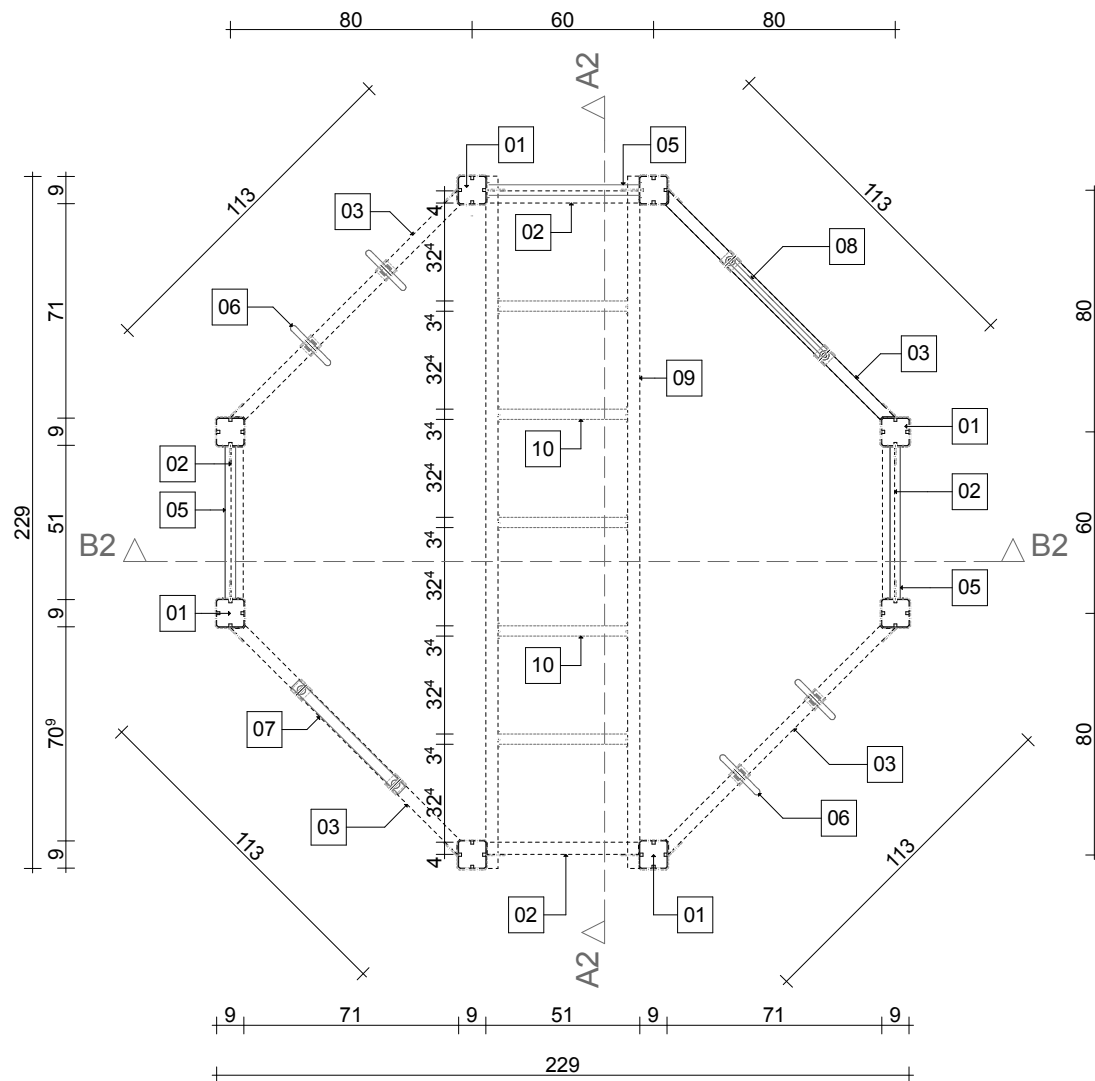
alaprajz m1:25
