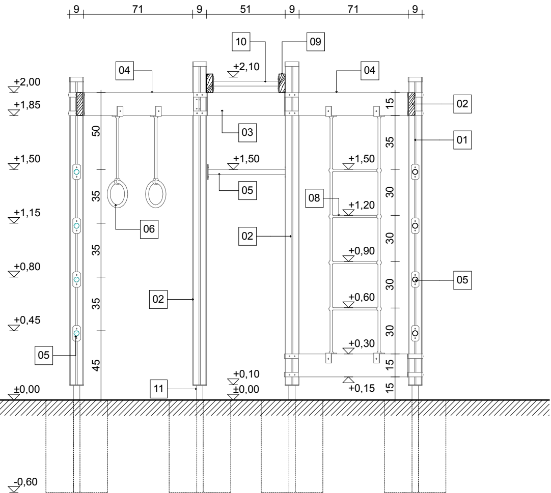
B-B metszet m1:25
