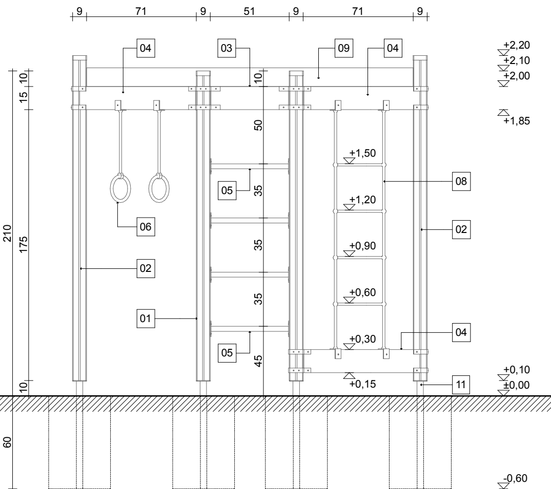
oldalnézet m1:25
