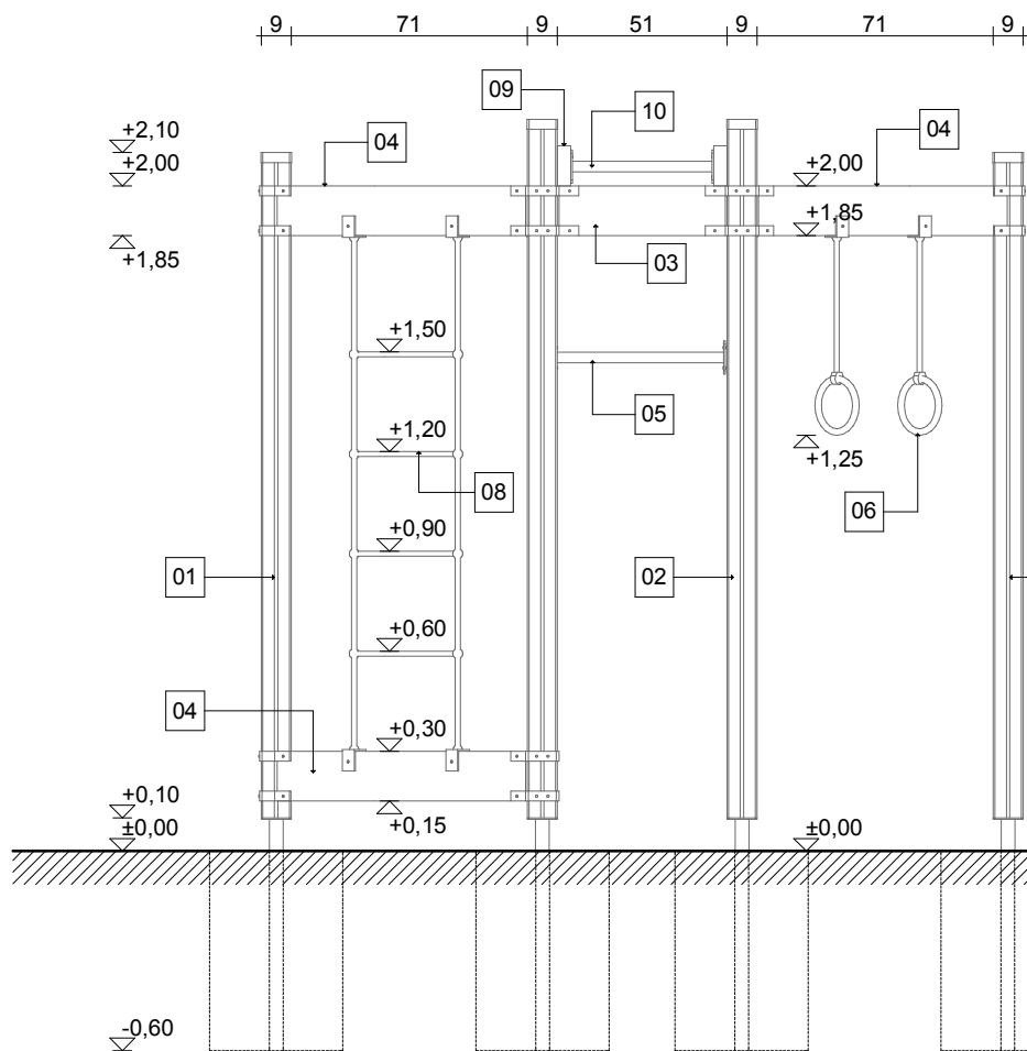
hátulnézet m1:25
