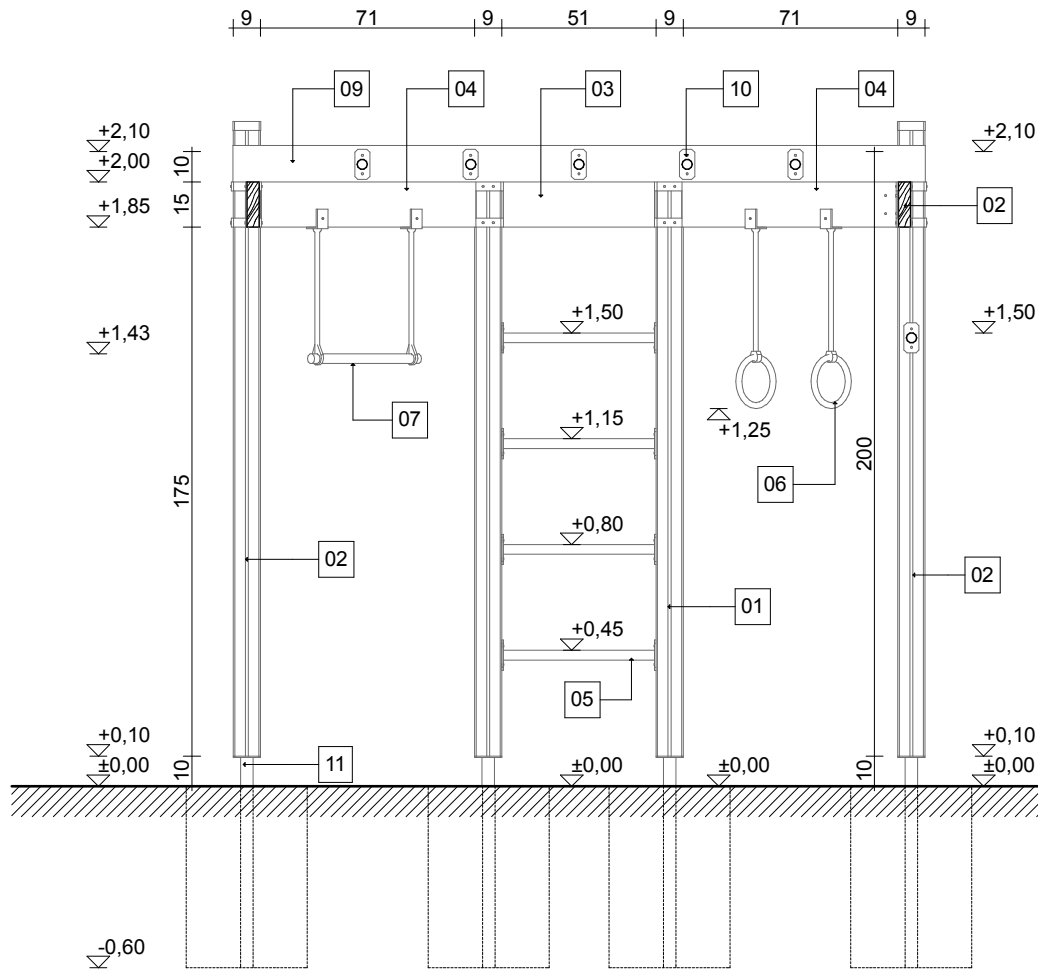
A-A metszet m1:25
