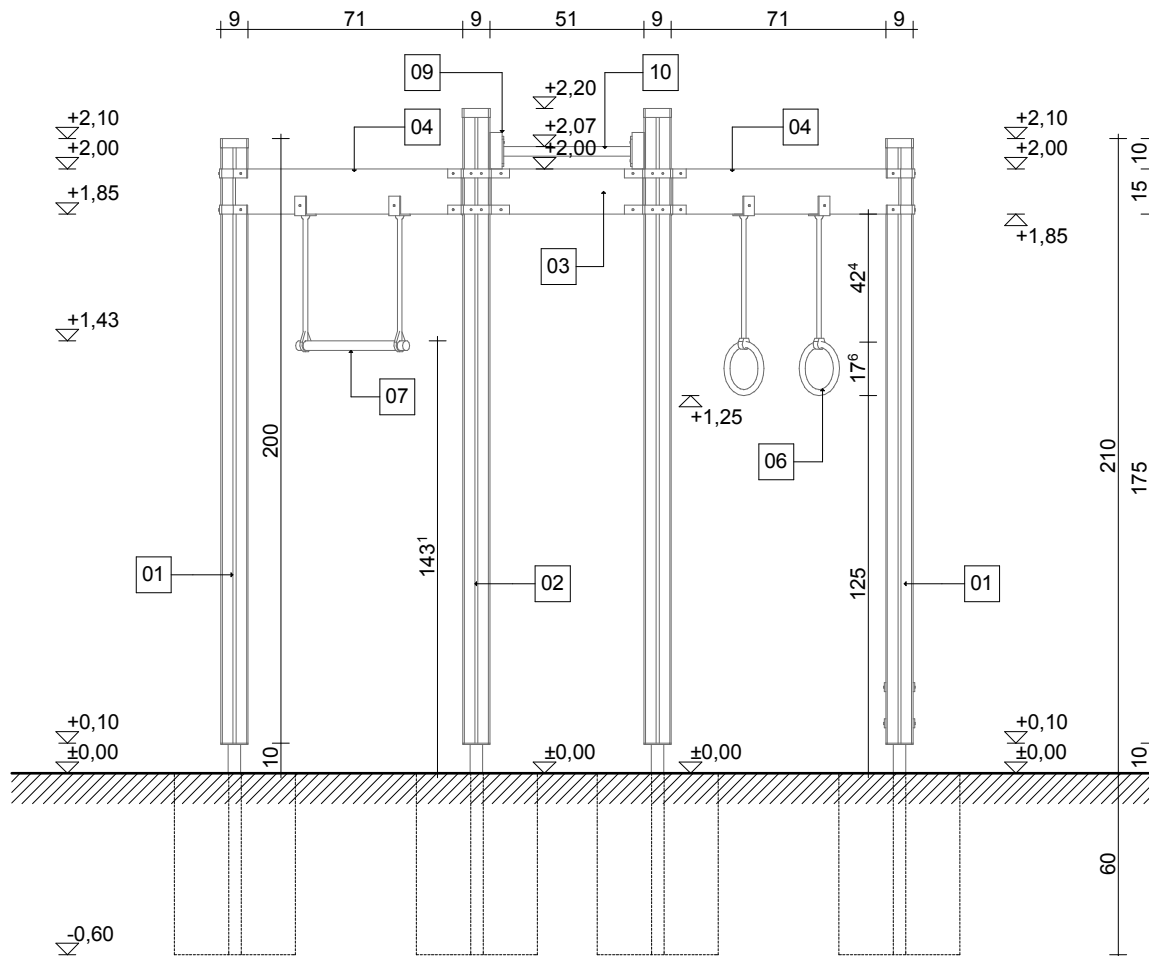
előlnézet m1:25
