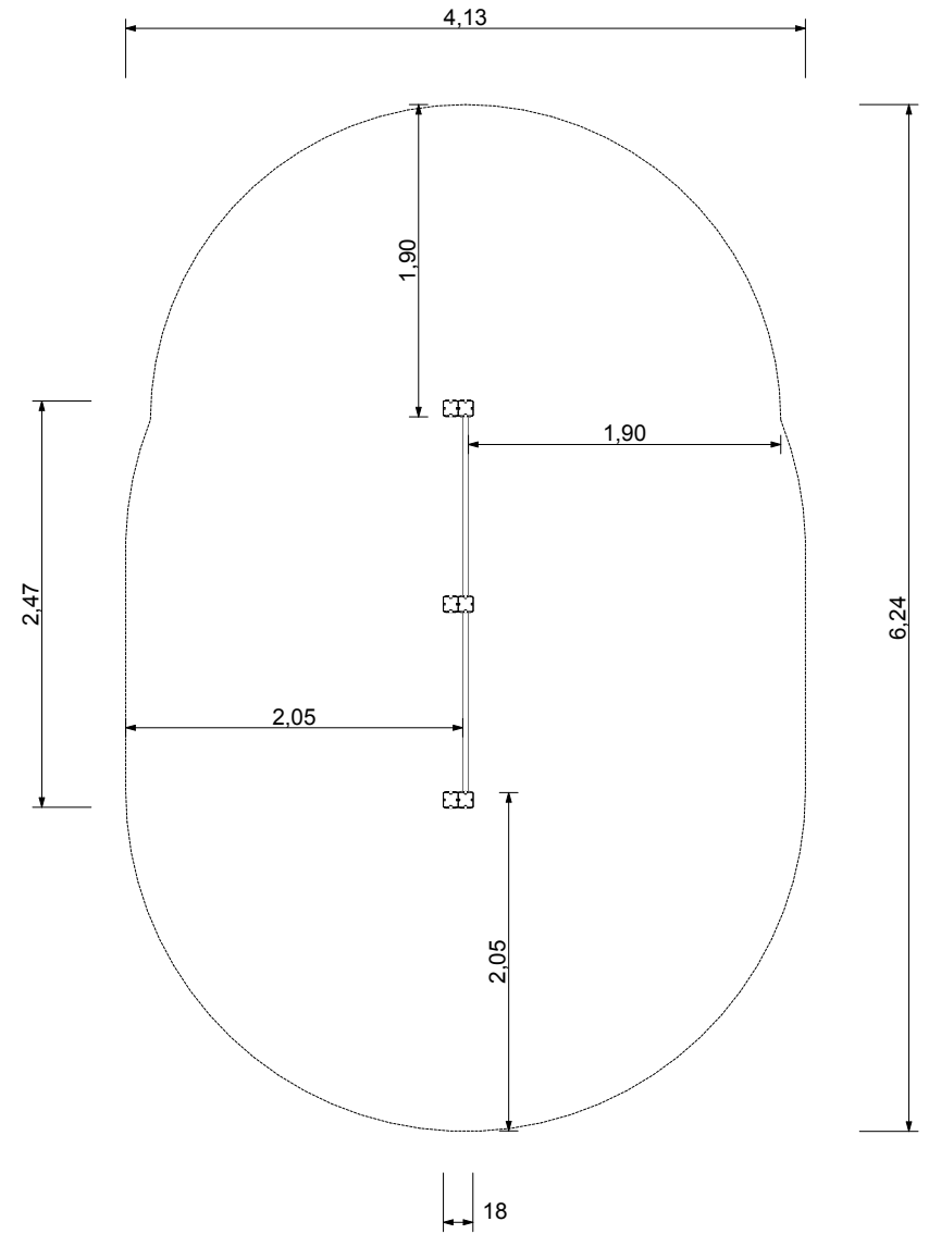
esési térkép m 1:50
