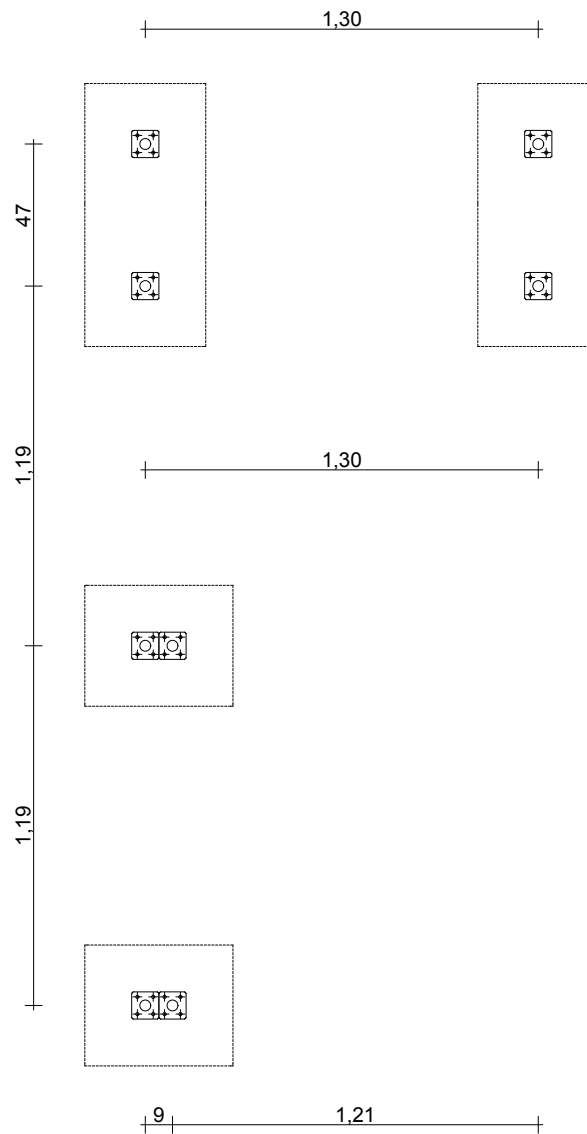
alapozási alaprész m 1:25
