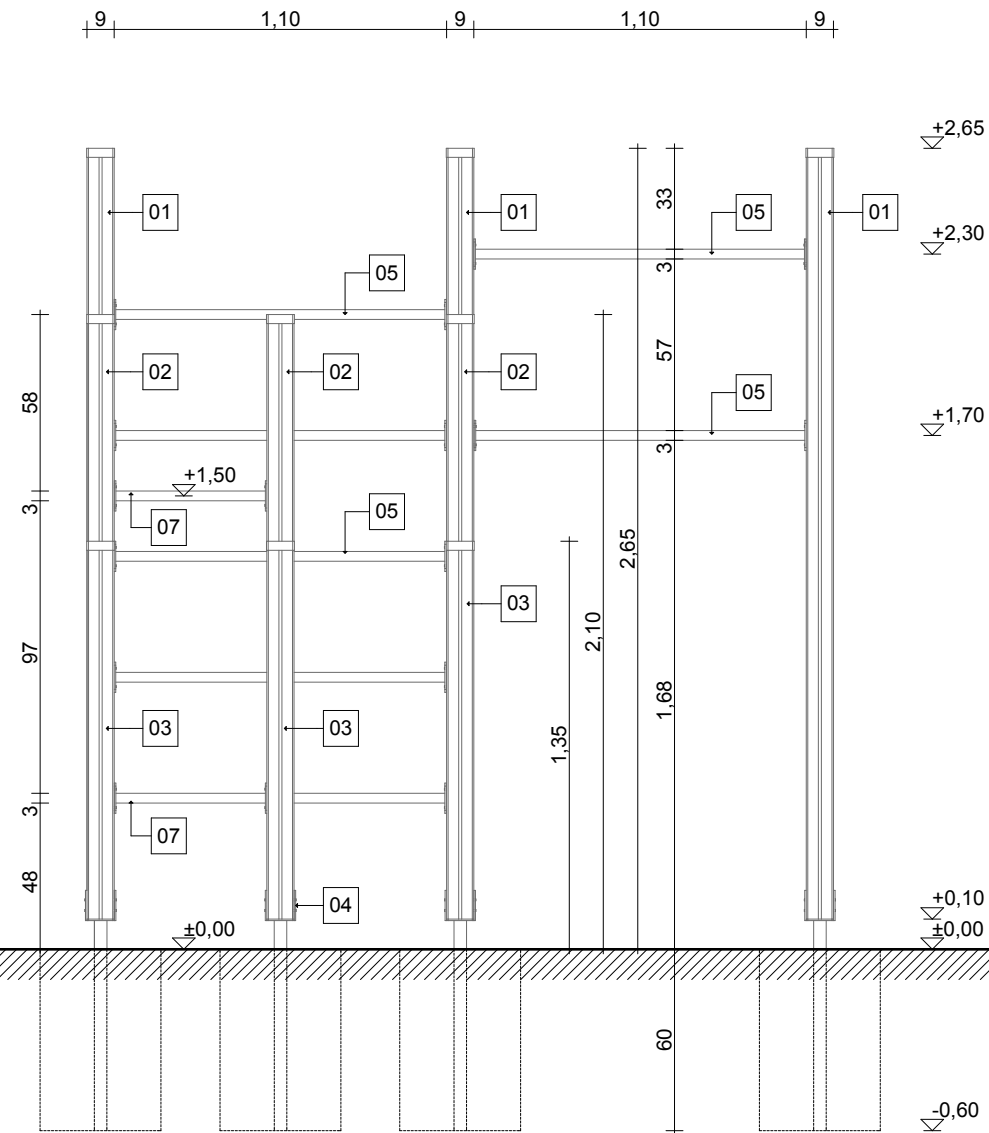
4. nézet m1:25
