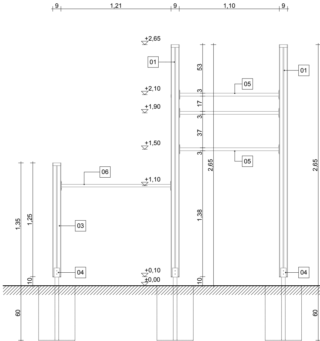
1. nézet m1:25
