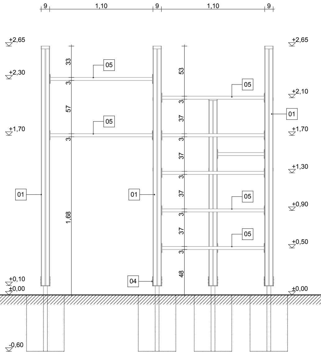
2. nézet m1:25
