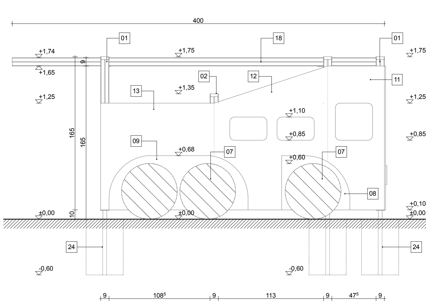
oldalnézet m1:25
