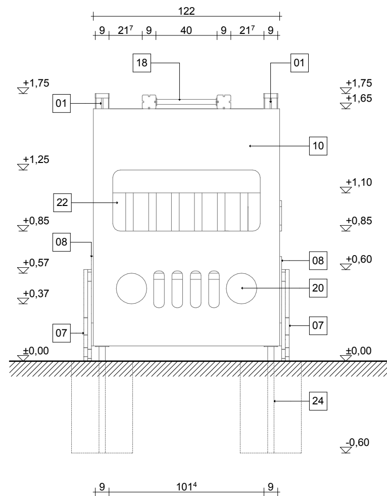
előlnézet m1:25
